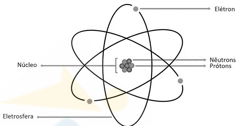
Figura 1 – Representação de modelo atômico
