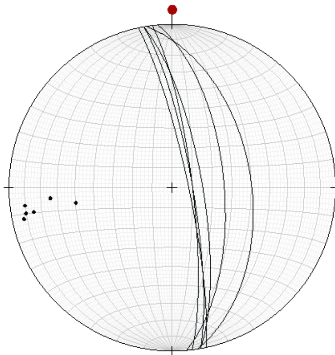
Figura 5. Estereograma dos veios de quartzo.
