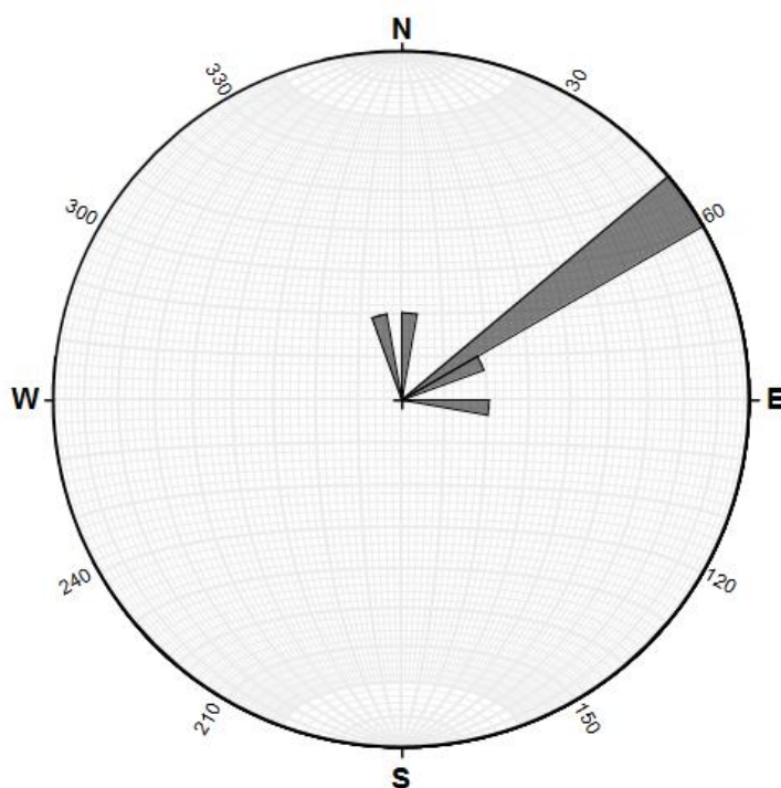
Figura 7. Diagrama de roseta com a principais fraturas que ocorrem no veio de quartzo.
