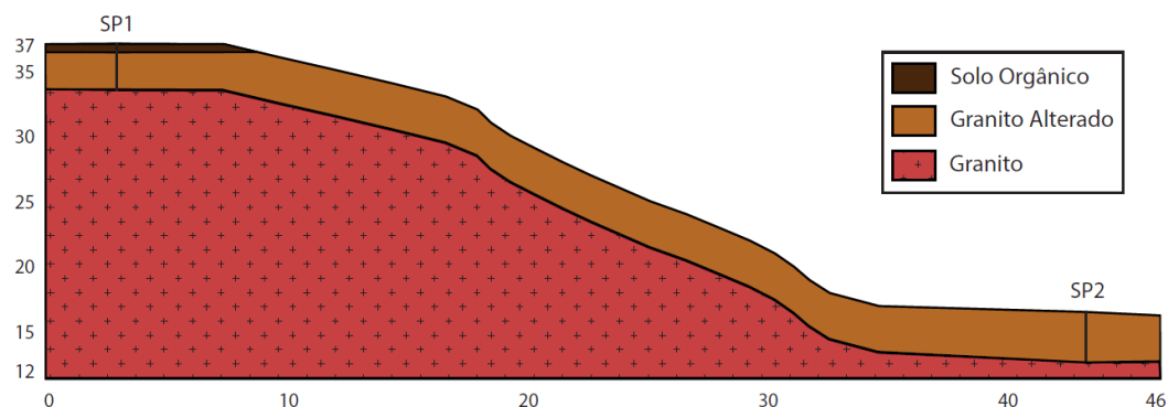
Figura 27. Seção entre as sondagens à percussão.
