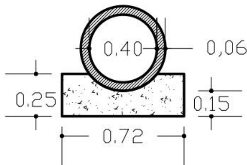
Bueiro Simples Tubular de Concreto – BSTC Ø 0,40m.
