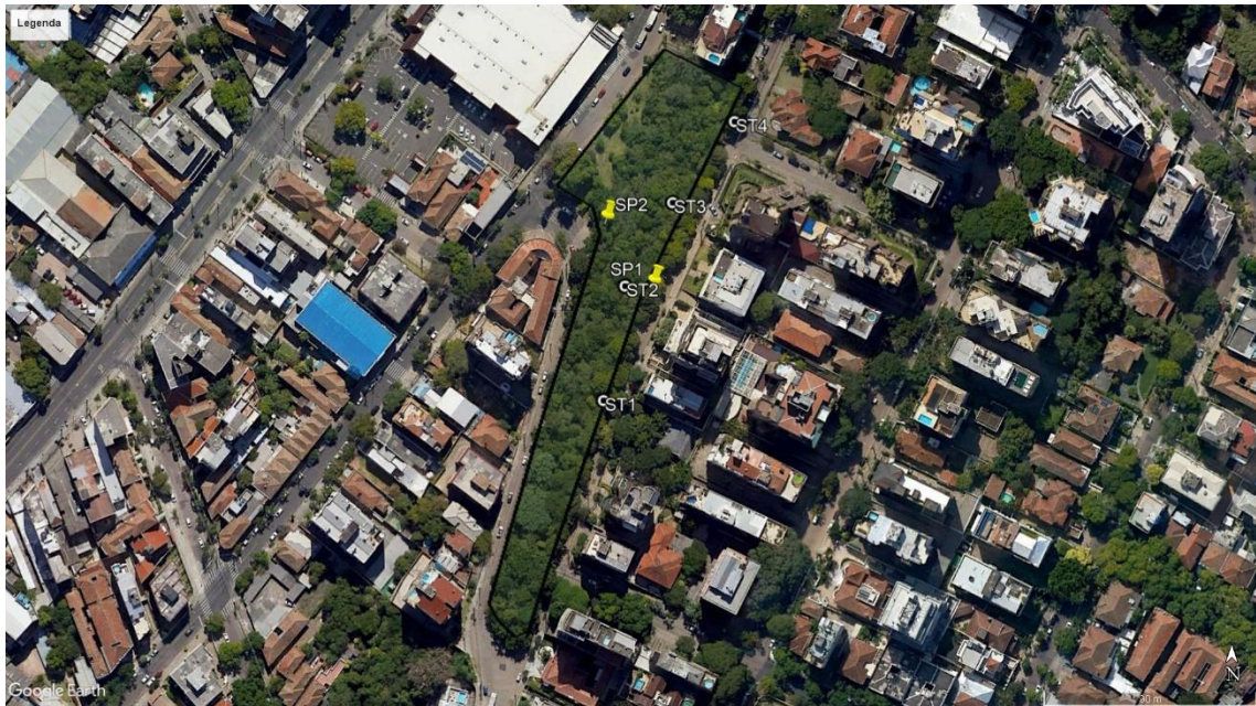
Figura 19. Disposição das sondagens na área de estudo
