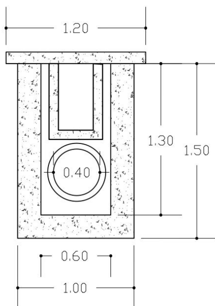
Caixa Coletora de Sarjeta (CCS)
