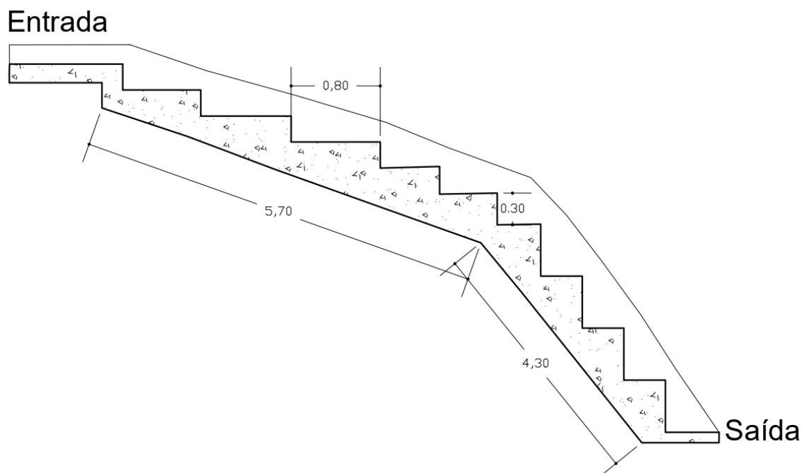
Descidas D'água em Degraus (DAD)
