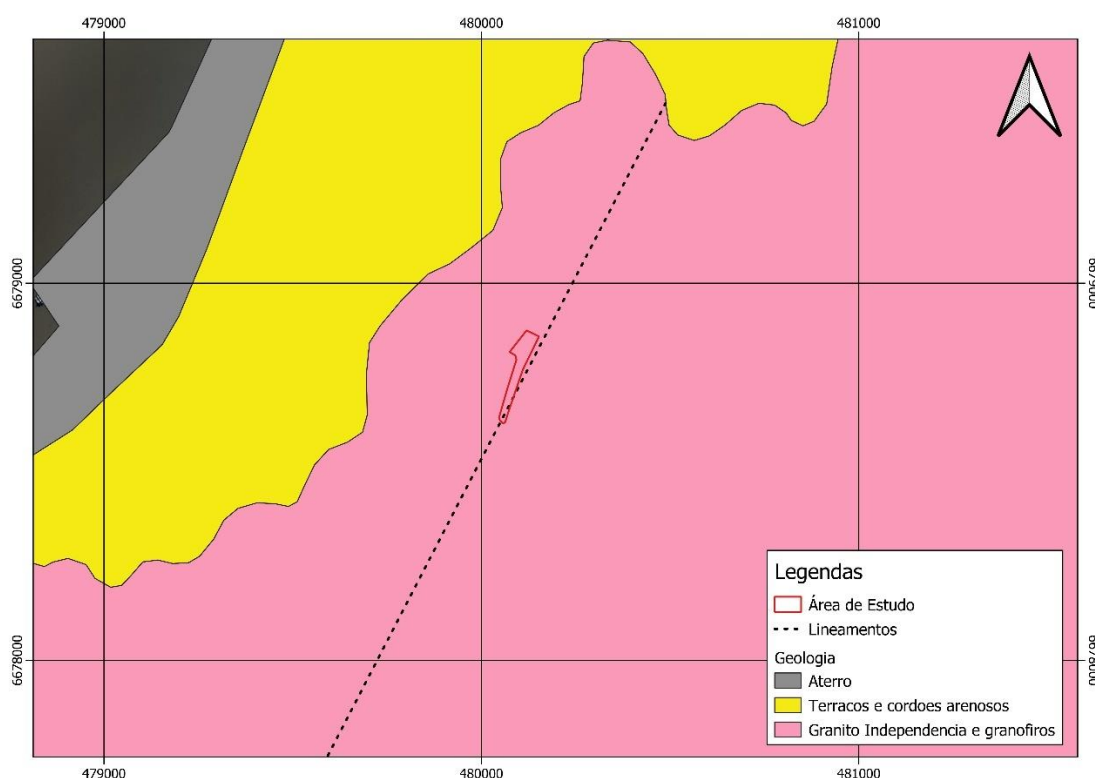
Figura 1 - Mapa geológico regional
