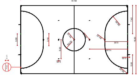
Pintura Demarcatória Futsal L = 178,00 m
