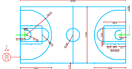
Pintura Demarcatória Basquete L = 243,20 m
