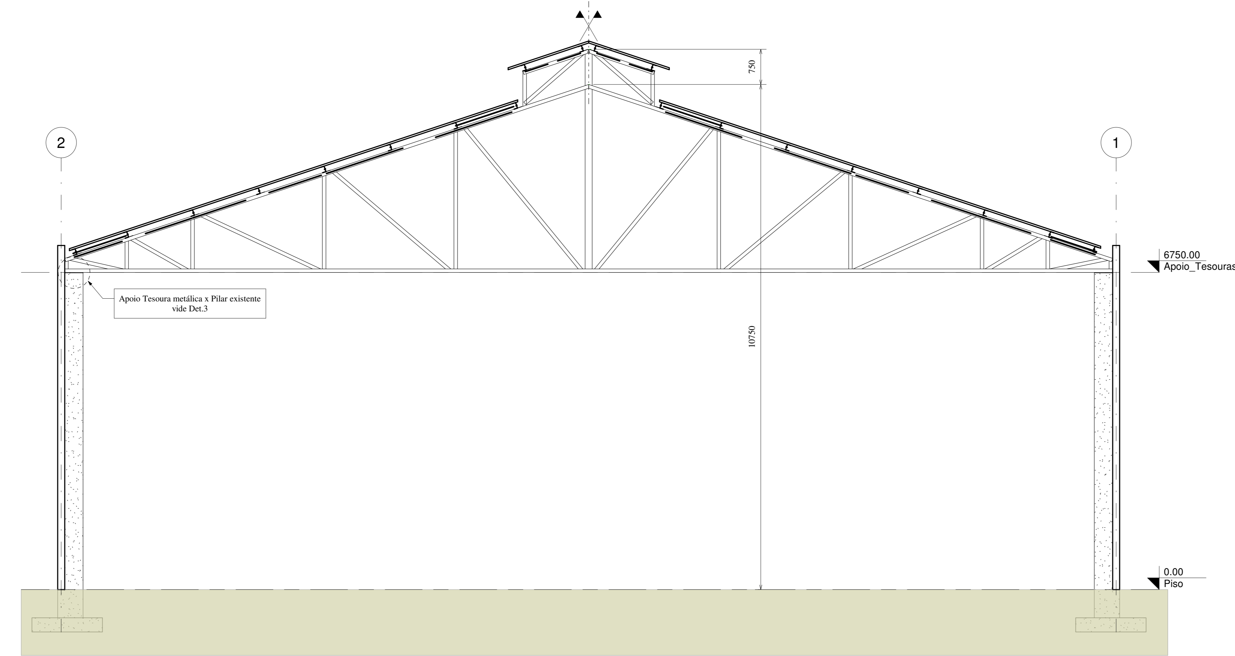
Corte C C 1 : 50
