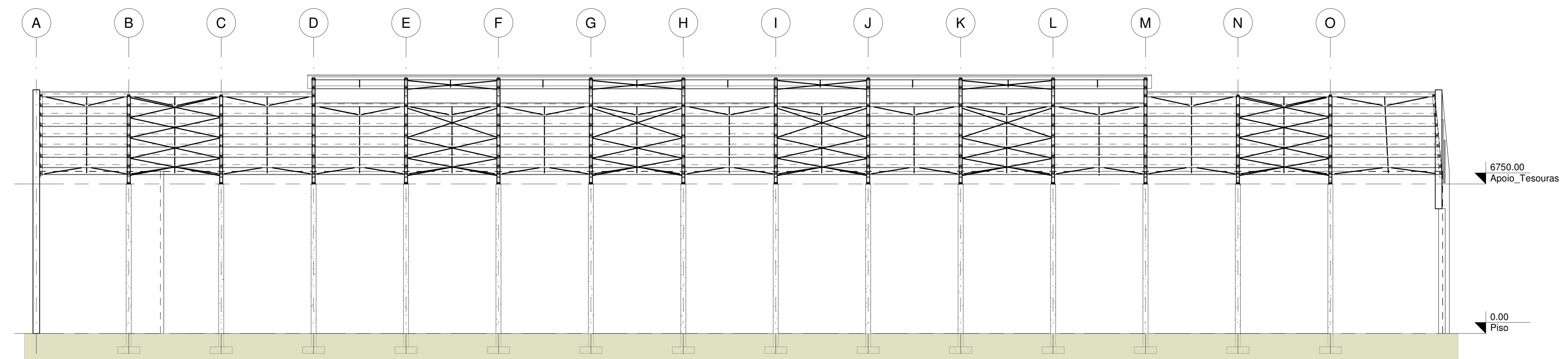
Corte D D 1 : 100
