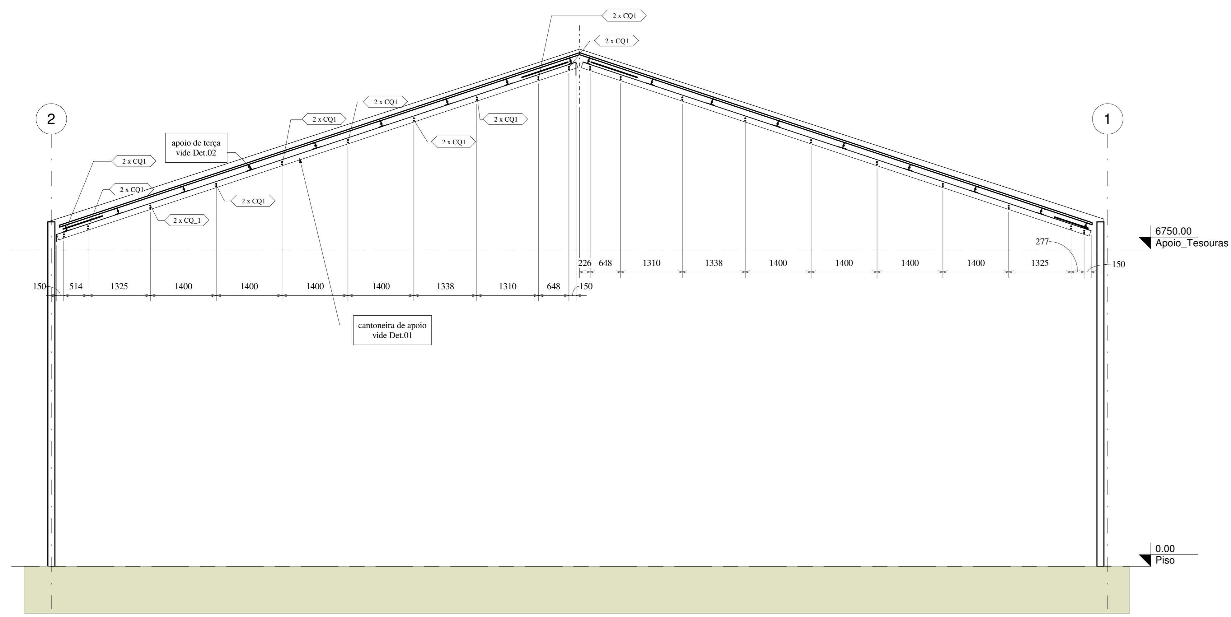
Corte AA 1 : 50
