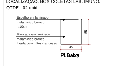
BANCADA BOX COLETAS - DET. 09 LOCALIZAÇÃO: BOX COLETAS LAB. IMUNO. QTDE - 02 und.
