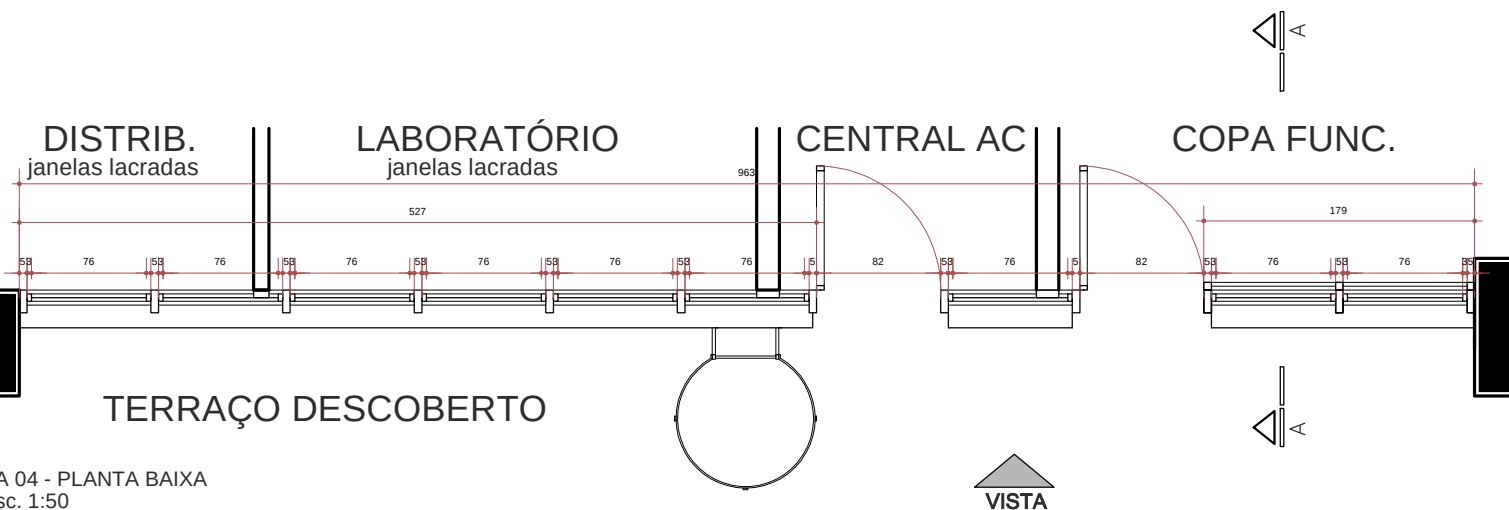
JA 04 - PLANTA BAIXA Esc. 1:50
