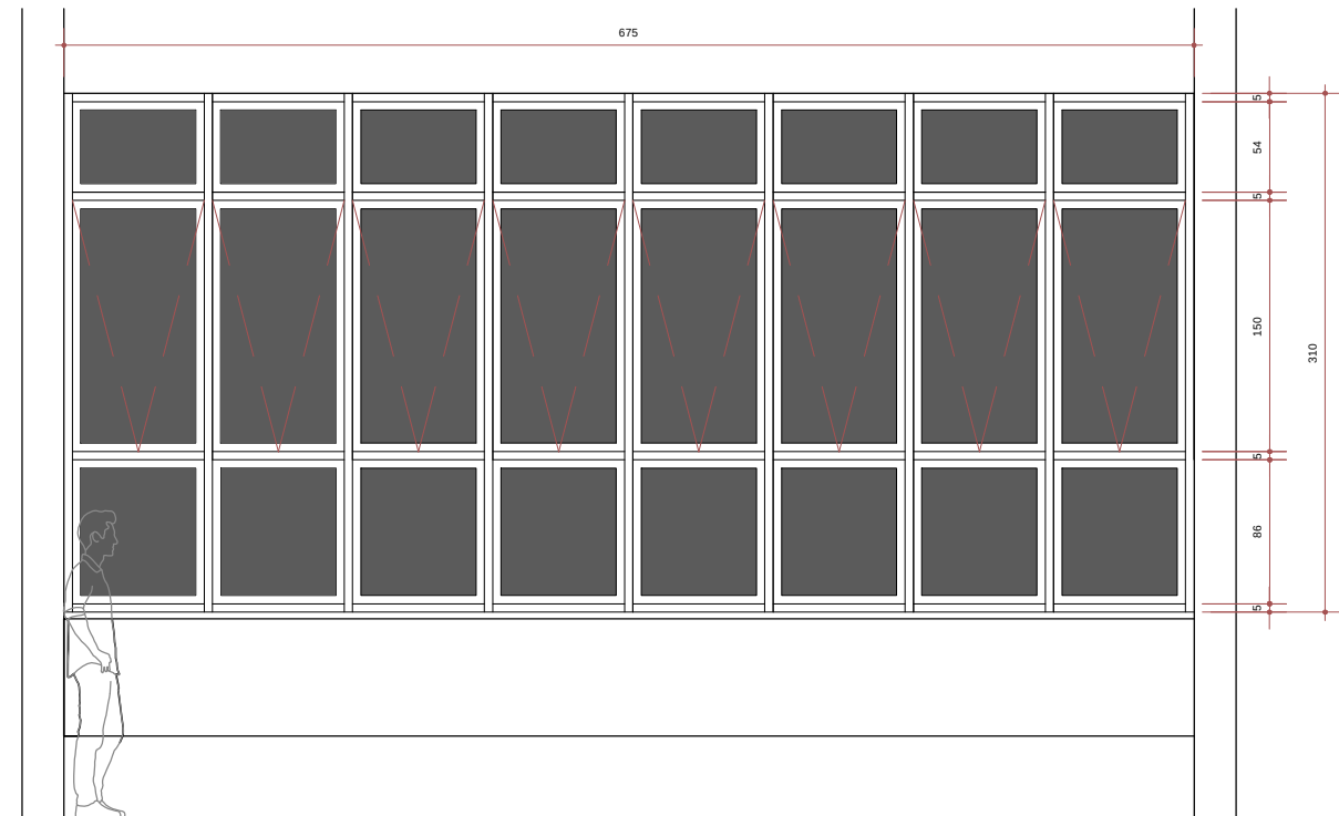
JA 01 - VISTA Esc. 1:50
