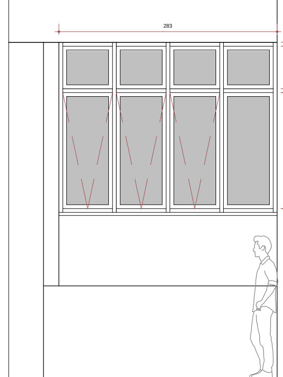
JA 03 - VISTA Esc. 1:50
