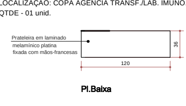
BANCADA COPA - DET. 10 LOCALIZAÇÃO: COPA AGÊNCIA TRANSF. LAB. IMUNO. QTDE - 01 und.
