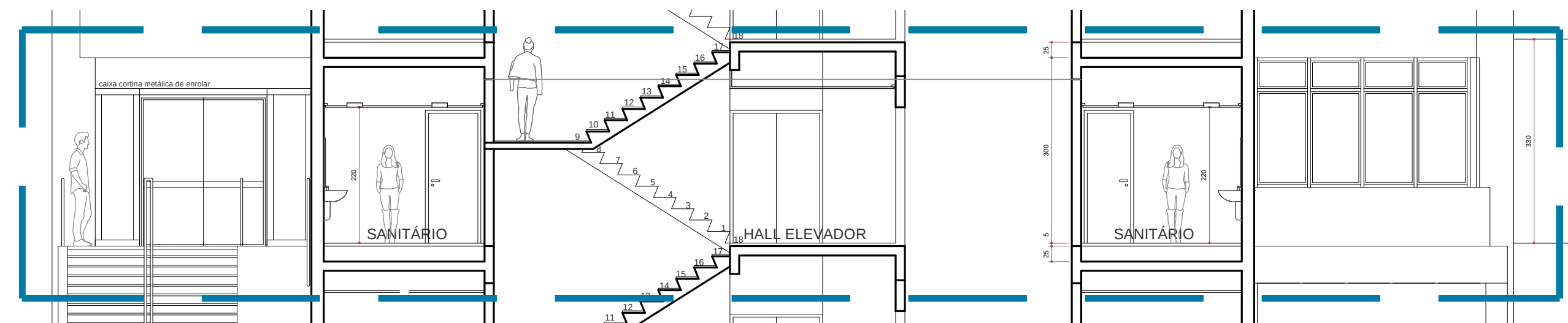
CORTE C-C Esc.1:75
