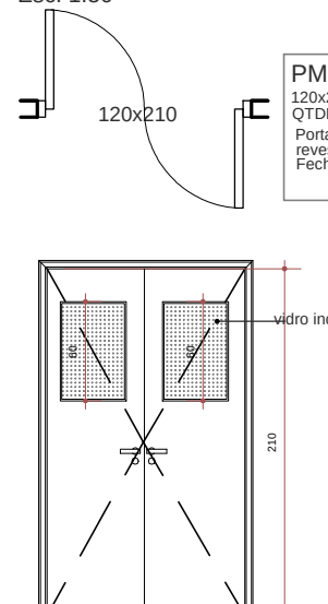
PM 03 - VISTA Esc. 1:50
