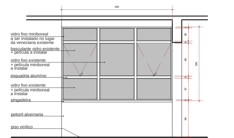
JA 06 EXISTENTE - VISTA Esc. 1:50
