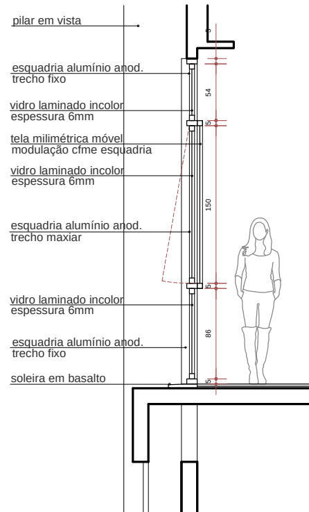
JA 01 - CORTE A-A Esc. 1:50
