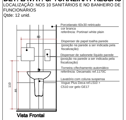
DET. LAVAT. C/ TORNEIRA PRESSÃO LOCALIZAÇÃO: NOS 10 SANITÁRIOS E NO BANHEIRO DE FUNCIONÁRIOS Qtde: 12 und.
