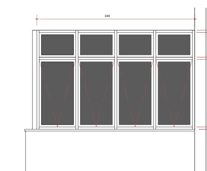
JA 05 - VISTA Esc. 1:50
