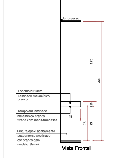
MÓVEL GUICHÊ RECEPÇÃO - DET. 1b LOCALIZAÇÃO: SAGUÃO DE ESPERA QTDE - 01 und.
