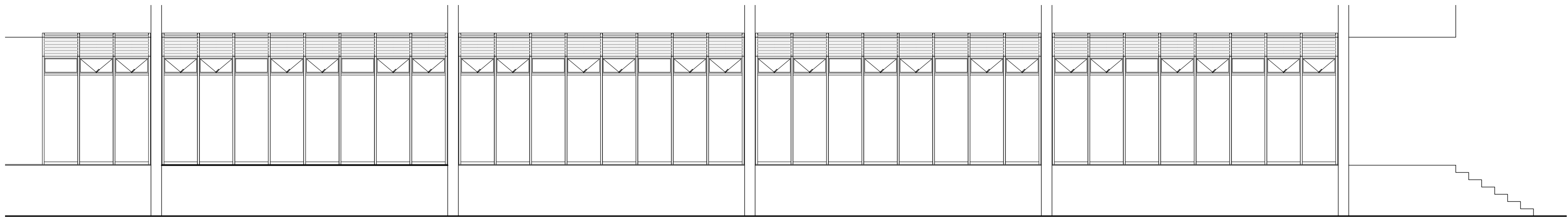
ELEVACÃO - MODULAÇÃO ESQUADRIA FACHADA Esc.1:75
