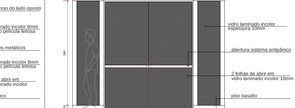
PV 04 - VISTA Esc. 1:50
