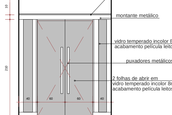
PV 02 - VISTA Esc. 1:50
