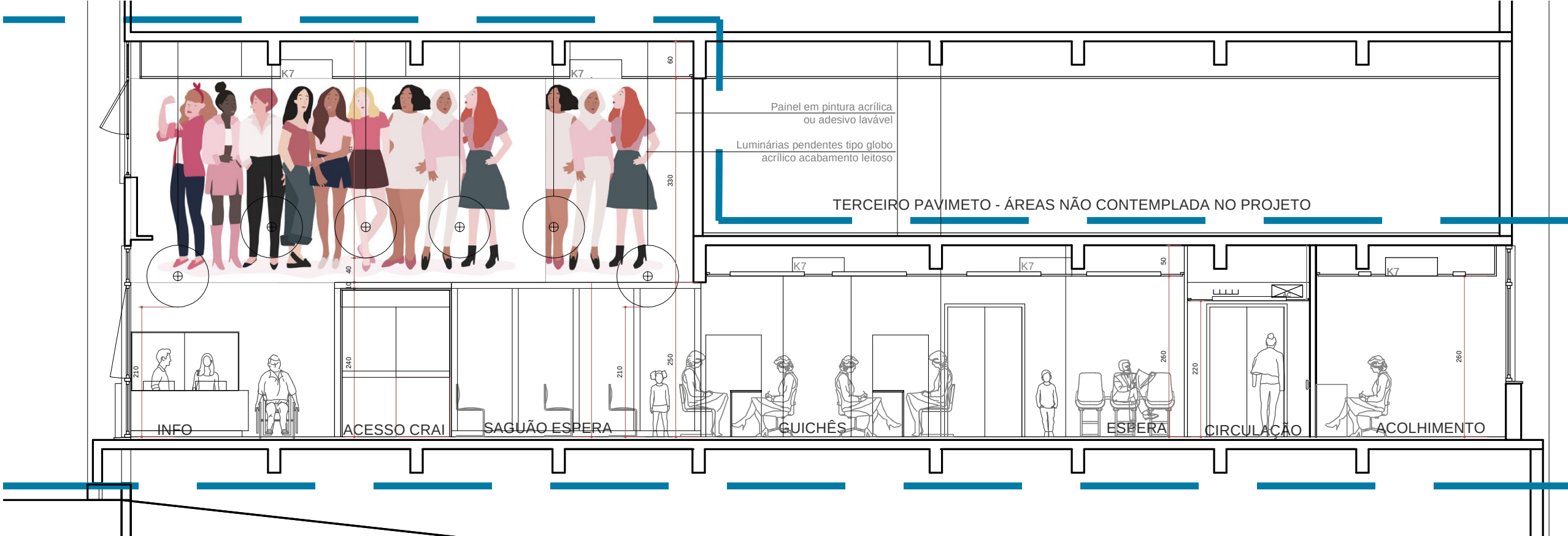
CORTE D-D Esc.1:75
