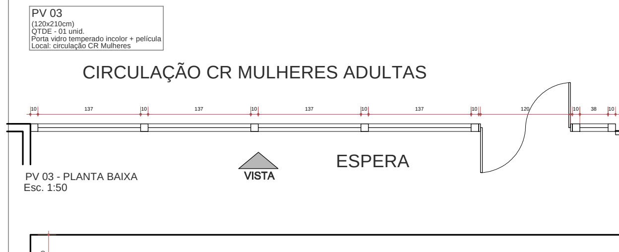
PV 03 - PLANTA BAIXA Esc. 1:50
