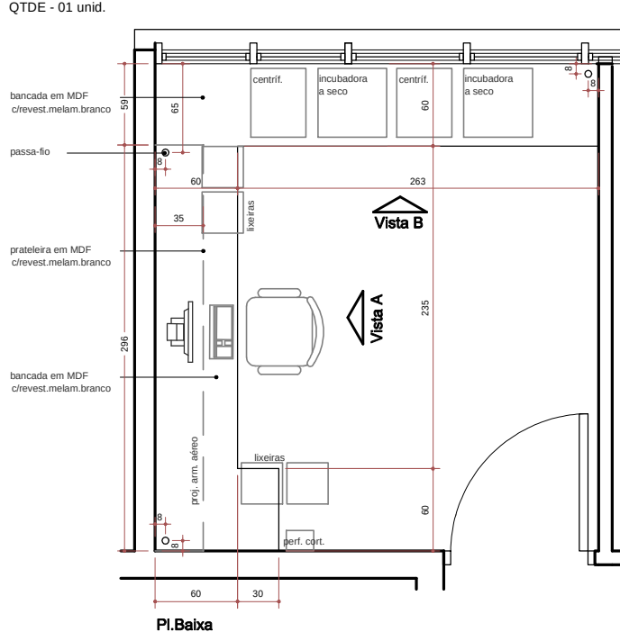
BANCADA E PRATELEIRA LABORATÓRIO IMUNOHEMATO - DET. 05 LOCALIZAÇÃO: LABORATÓRIO IMUNOHEMATO QTDE - 01 und.
