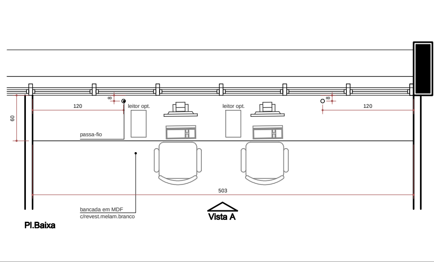
BANCADA E PRATELEIRA LABORATÓRIO IMUNOHEMATO - DET. 05 LOCALIZAÇÃO: LABORATÓRIO IMUNOHEMATO QTDE - 01 und.
