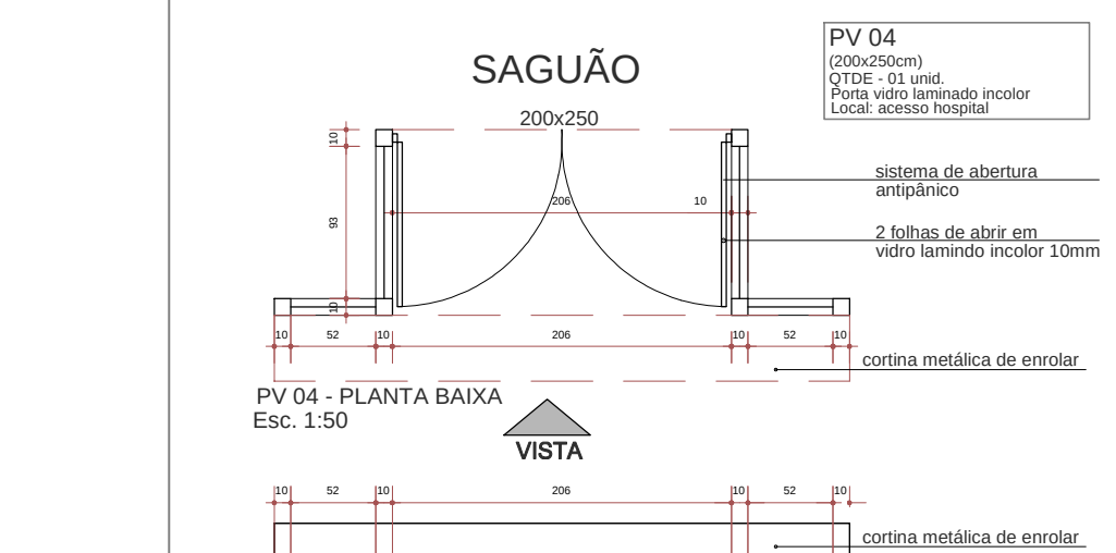
PV 04 - PLANTA BAIXA Esc. 1:50
