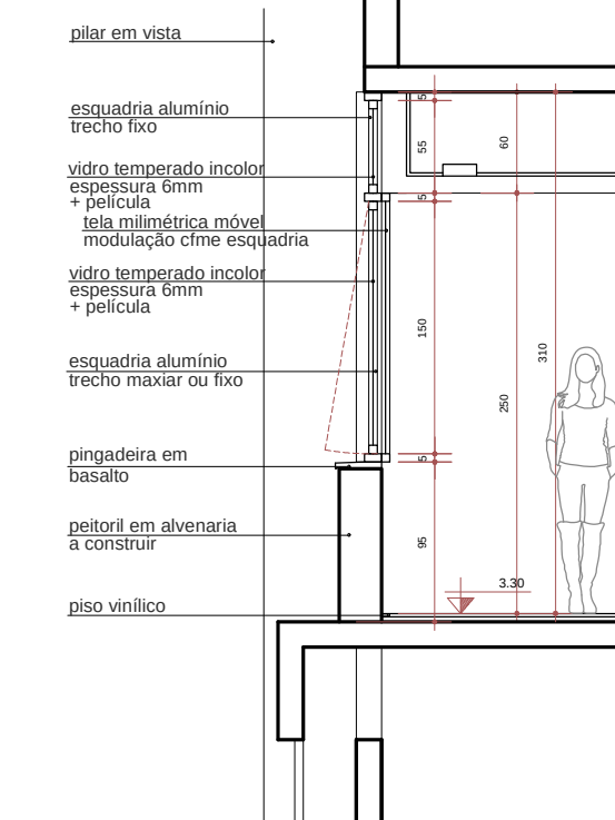
JA 02 - CORTE A-A Esc. 1:50
