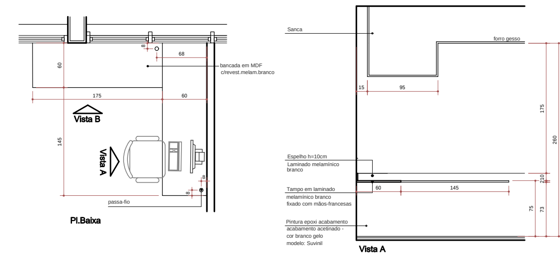
BANCADA DISTRIBUIÇÃO/COMPATIBILIZAÇÃO - DET. 06 LOCALIZAÇÃO: SALA DE DIST.COMPAT. AGÊNCIA TRANSF. QTDE - 01 und.
