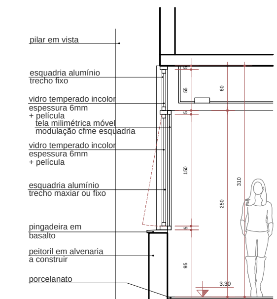
JA 04 - CORTE A-A Esc. 1:50
