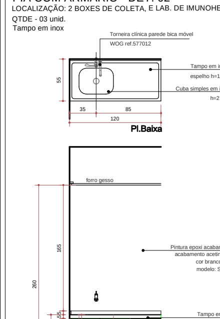
PIA COM ARMÁRIO - DET. 02 LOCALIZAÇÃO: 2 BOXES DE COLETA E LAB. DE IMUNO. QTDE - 03 und. Tampo em inox
