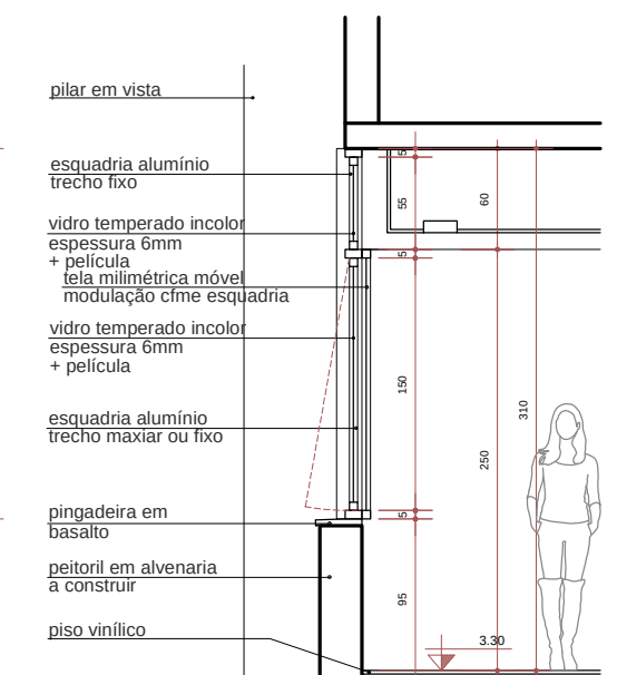
JA 05 - CORTE A-A Esc. 1:50
