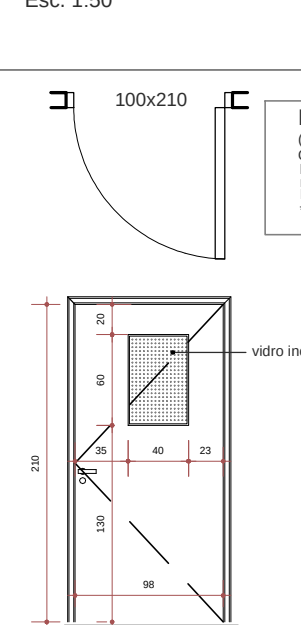
PM 02 - VISTA Esc. 1:50
