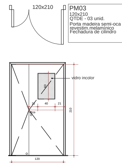
PM 03 - PLANTA BAIXA Esc. 1:50
