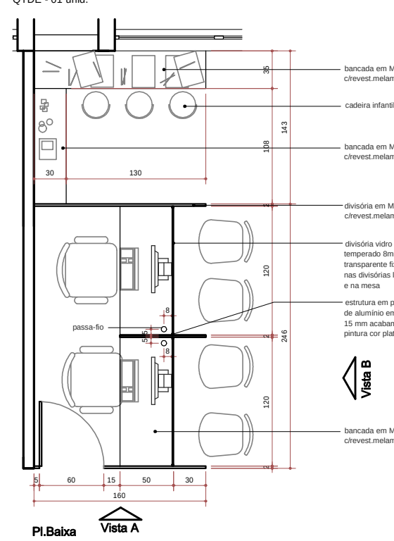
GUICHÊS E BANCADA ESPAÇO LÚDICO - DET. 11 LOCALIZAÇÃO: RECEPÇÃO CRAI QTDE - 01 und.
