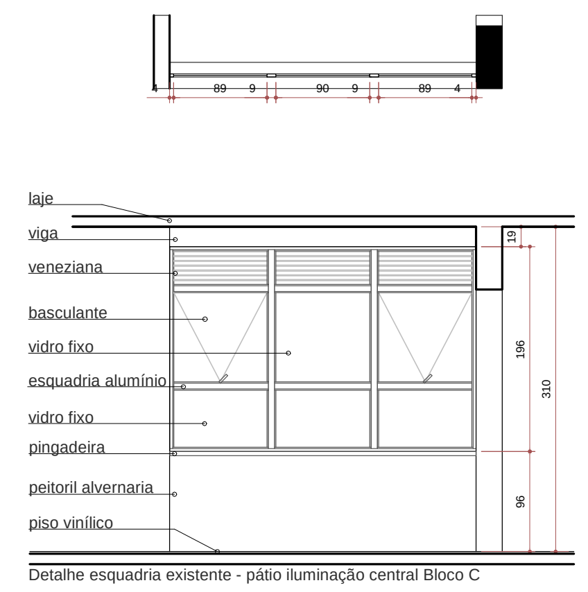
DET.MODULAÇÃO ESQUADRIA PÁTIO CENTRAL Esc.1:75
