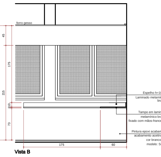
BANCADA COPA/ESTAR - DET. 08 LOCALIZAÇÃO: COPA/ESTAR FUNC. CRAI QTDE - 02 und.
