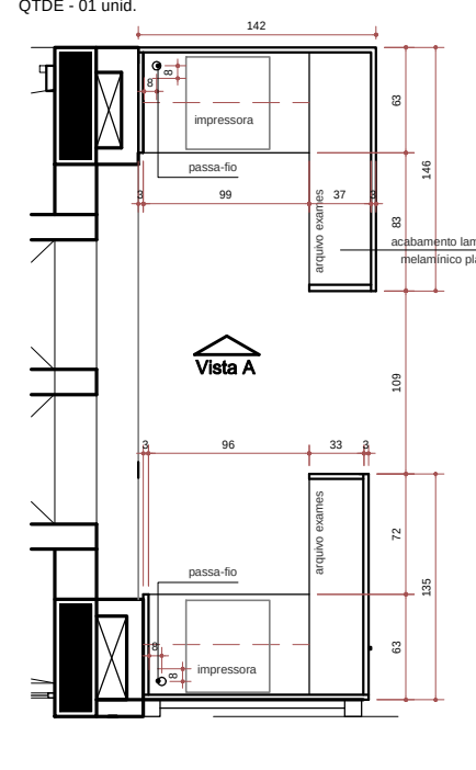
MÓVEL GUICHÊ RECEPÇÃO - DET. 1b LOCALIZAÇÃO: SAGUÃO DE ESPERA QTDE - 01 und.
