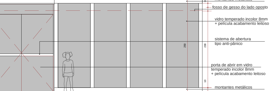
PV 01 - VISTA Esc. 1:50
