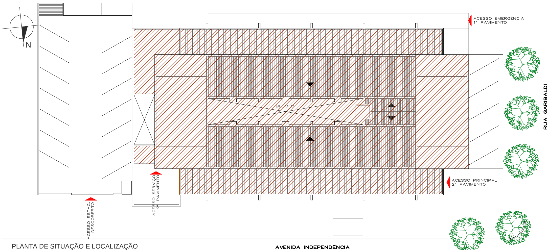
PLANTA DE SITUAÇÃO E LOCALIZAÇÃO Esc.1:250 ÁREA CONTEMPLADA NO PROJETO
