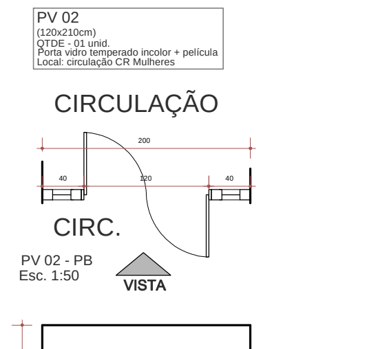
PV 02 - PLANTA BAIXA Esc. 1:50
