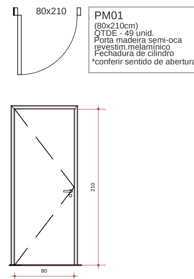
PM 01 - PLANTA BAIXA Esc. 1:50
